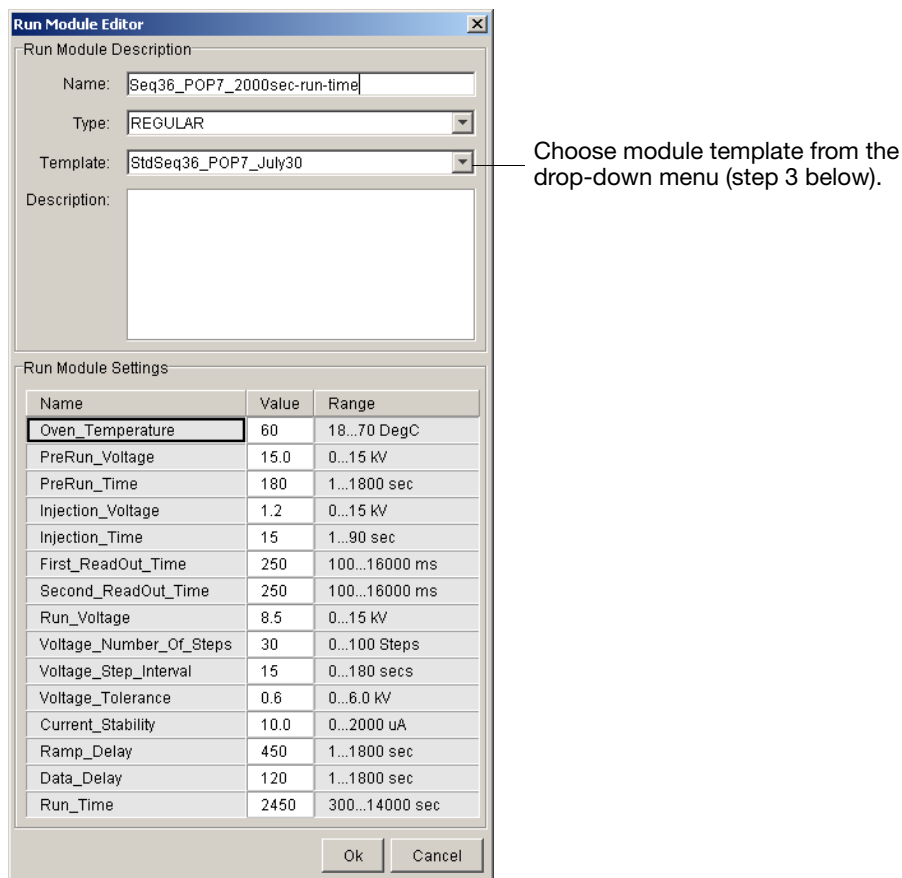
Figure 1-43 Customize Run Module Parameters
